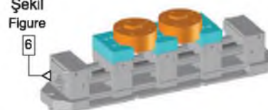
İş parçalarının kendi arasında 2mm kadar ölçü farkını içine sindiren mekanizma Sabit çene referanslı merkezden dışa bağlama şekli Figure based on fixed jaw clamping from centre in outward
