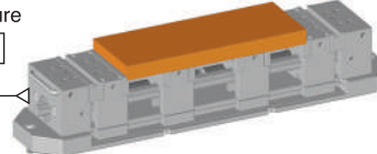
Gezer paraleller üzerinde ince iş parçası bağlama şekli Figure clamping thin workpiece on motion parallels
