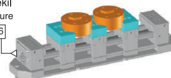
Yumuşak ayak ile bağlama şekli Figure clamping with soft legs
